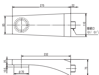
接続口25A/32A
