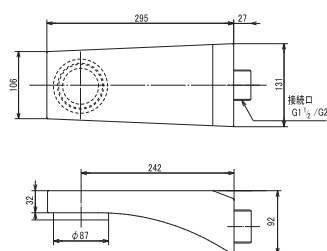
接続口40A/50A
