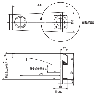
接続口25A/32A
