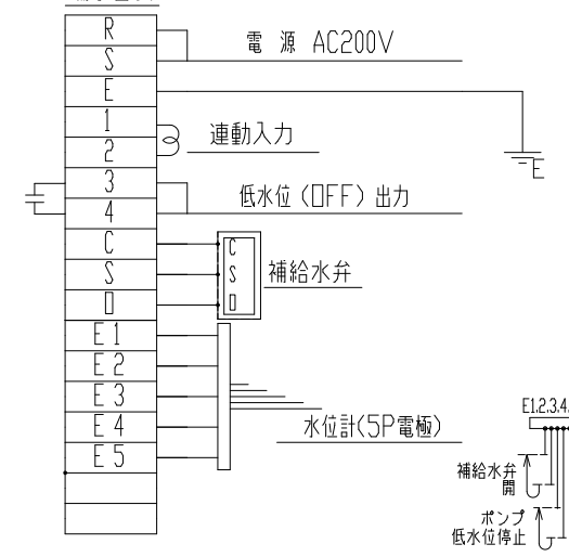
端子台表
