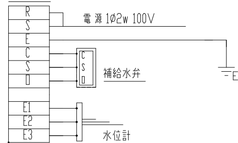
端子台表
